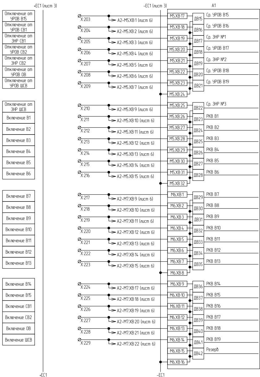
Рисунок В.4 – Схема электрическая принципиальная (часть 4)
