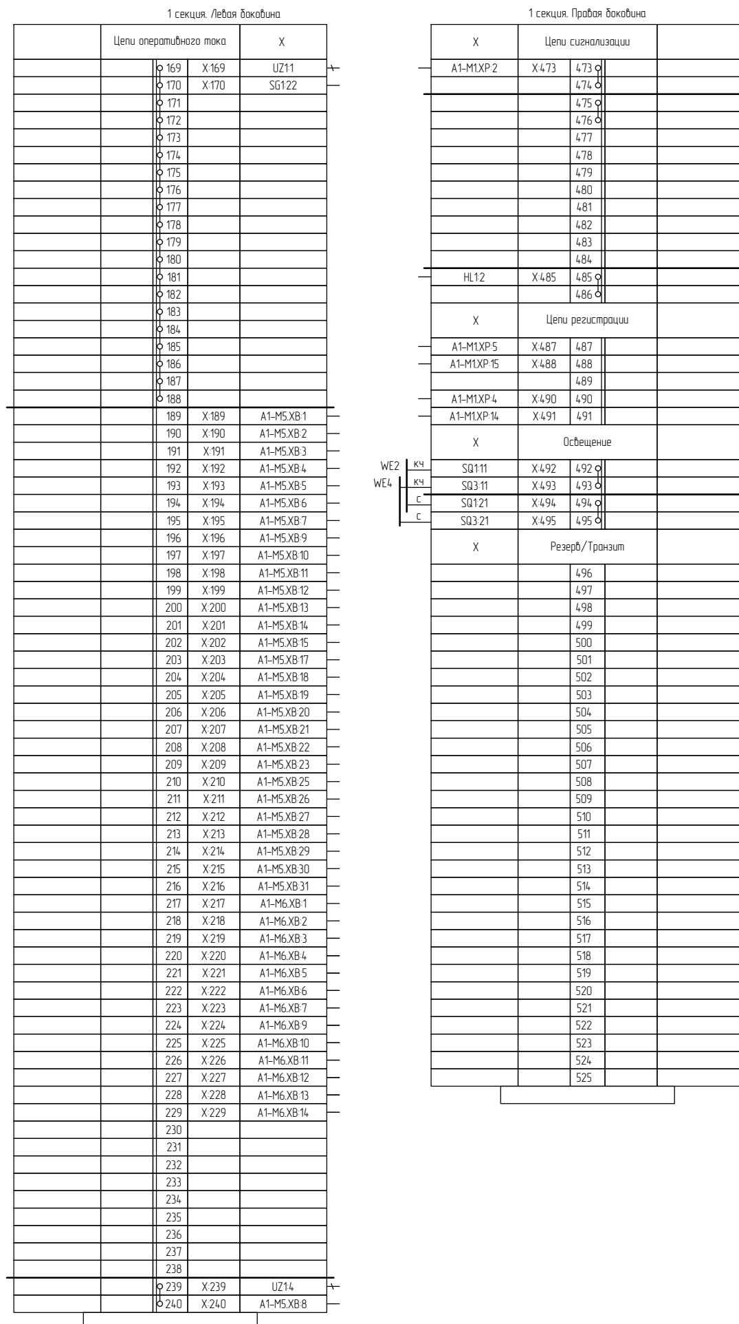
Рисунок Г.5 – Схема электрическая соединений рядов зажимов (часть 5)
