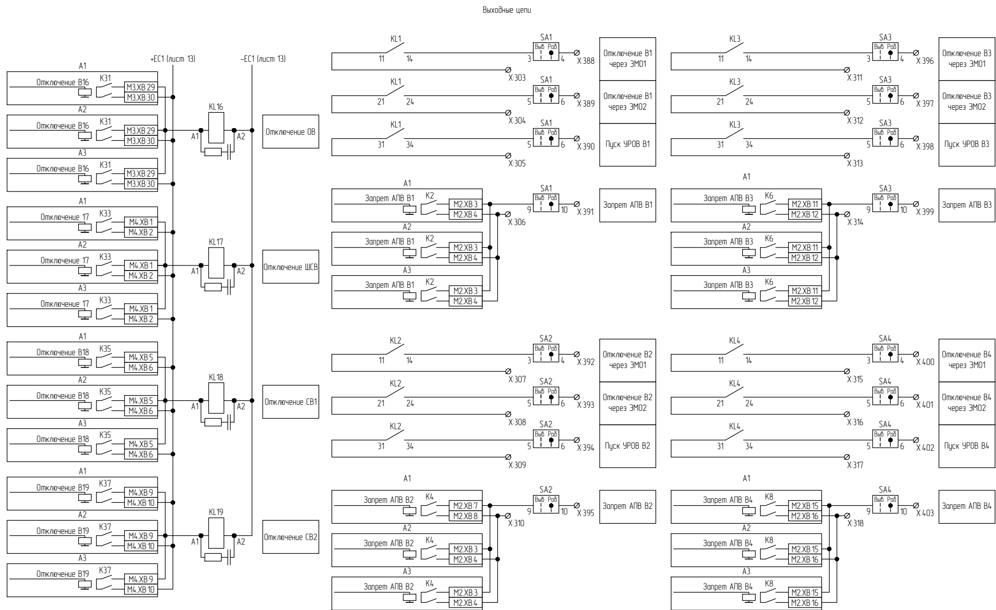
Рисунок В.14 – Схема электрическая принципиальная (часть 14)
