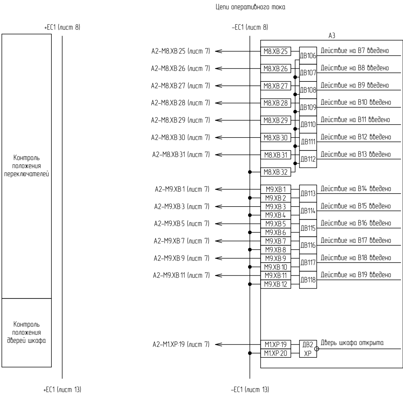
Рисунок В.9 – Схема электрическая принципиальная (часть 9)
