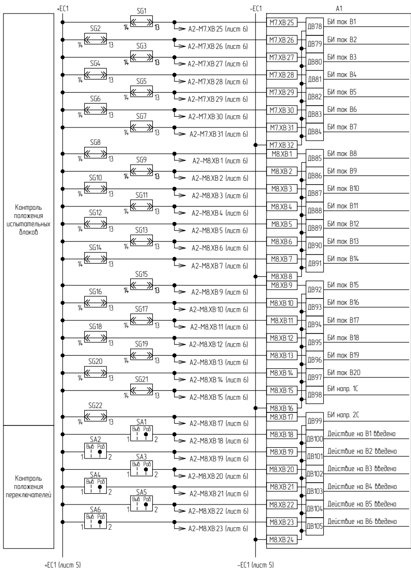
Цели оперативного тока
