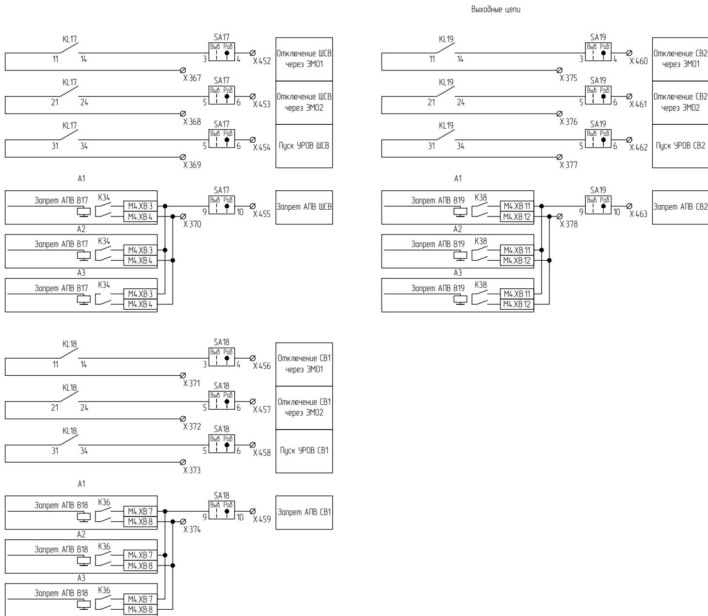
Рисунок В.17 – Схема электрическая принципиальная (часть 17)
